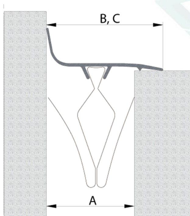
FIJACIÓN**
